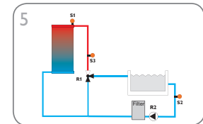
Sistema solar para calentamiento de piscina con operación de filtración (pág. 13)
