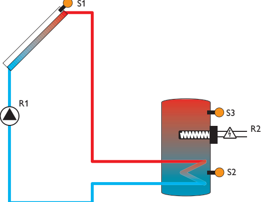
Sistema 1, variante b sistema de energía solar estándar con 1 acumulador y calentamiento auxiliar eléctrico
