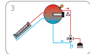
Sistema de termosifón (página 11)
