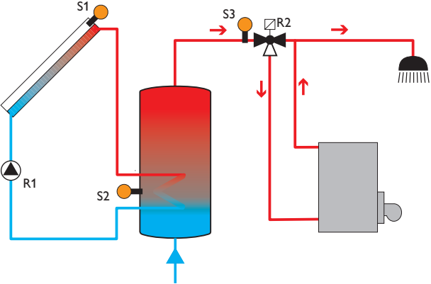
Sistema 1, variante a: sistema de energía solar estándar con 1 acumulador y calentamiento auxiliar
